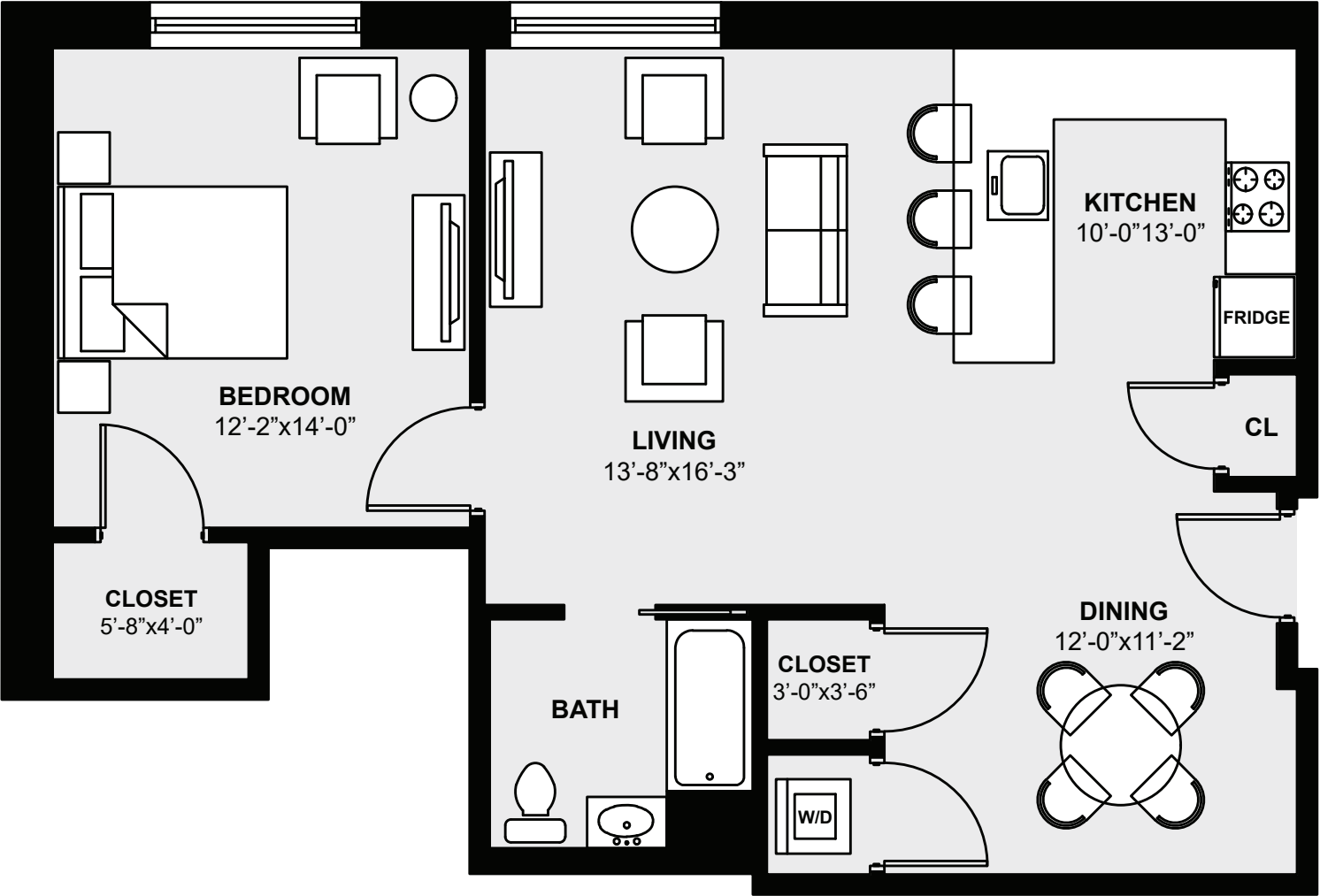
UNIT 205 782 SF.
